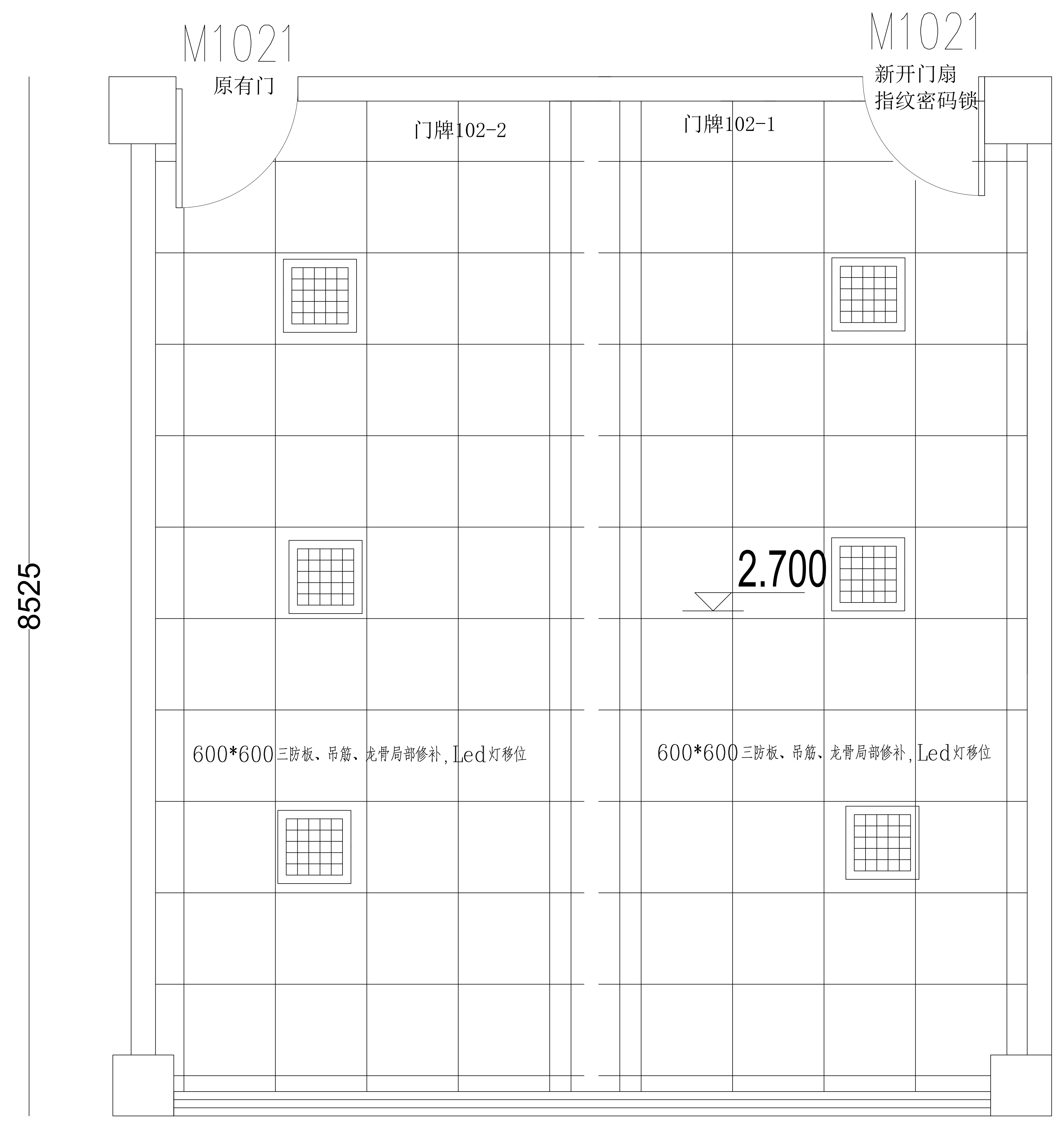
吊顶面布置图
