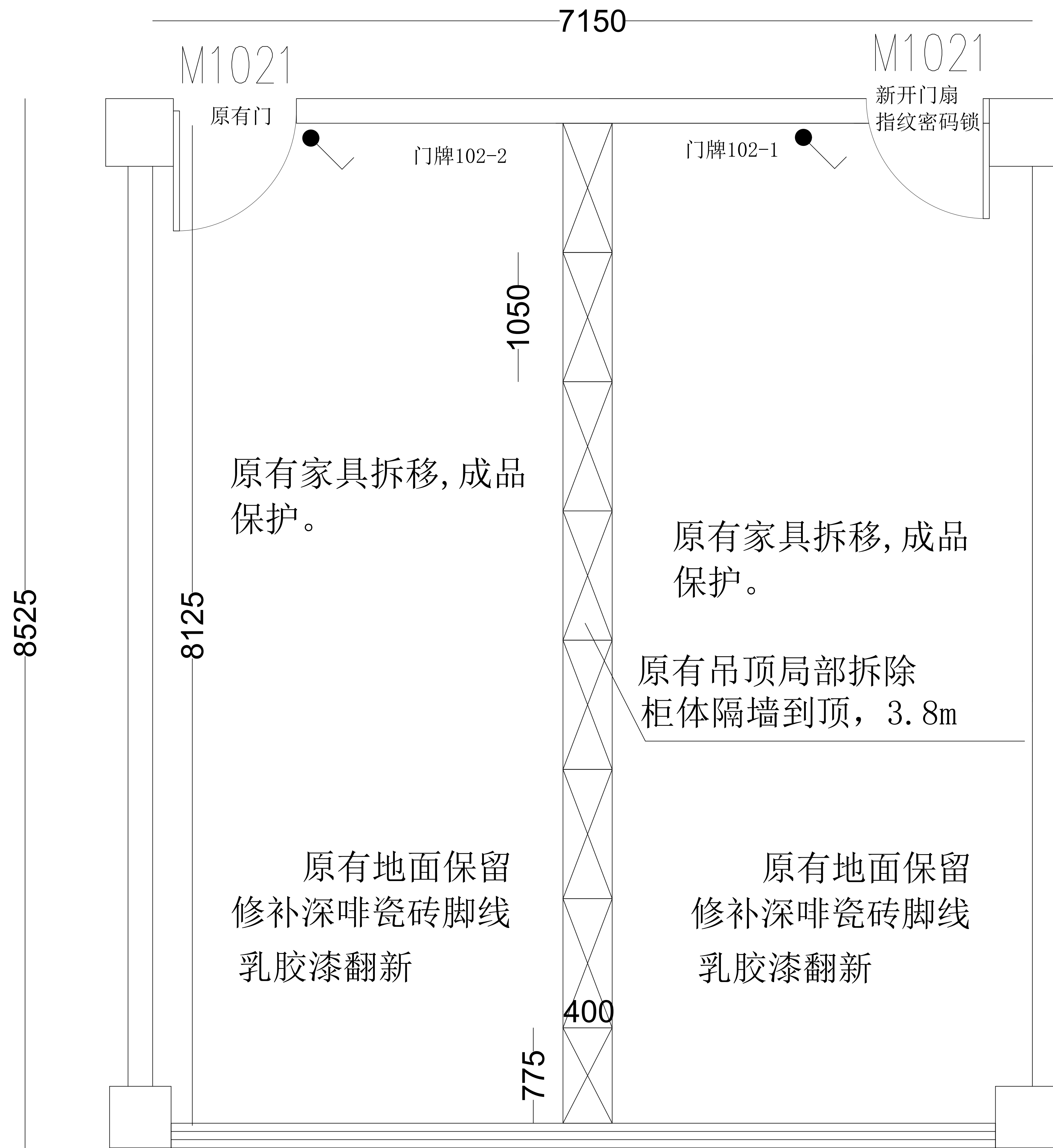
结构改造图
