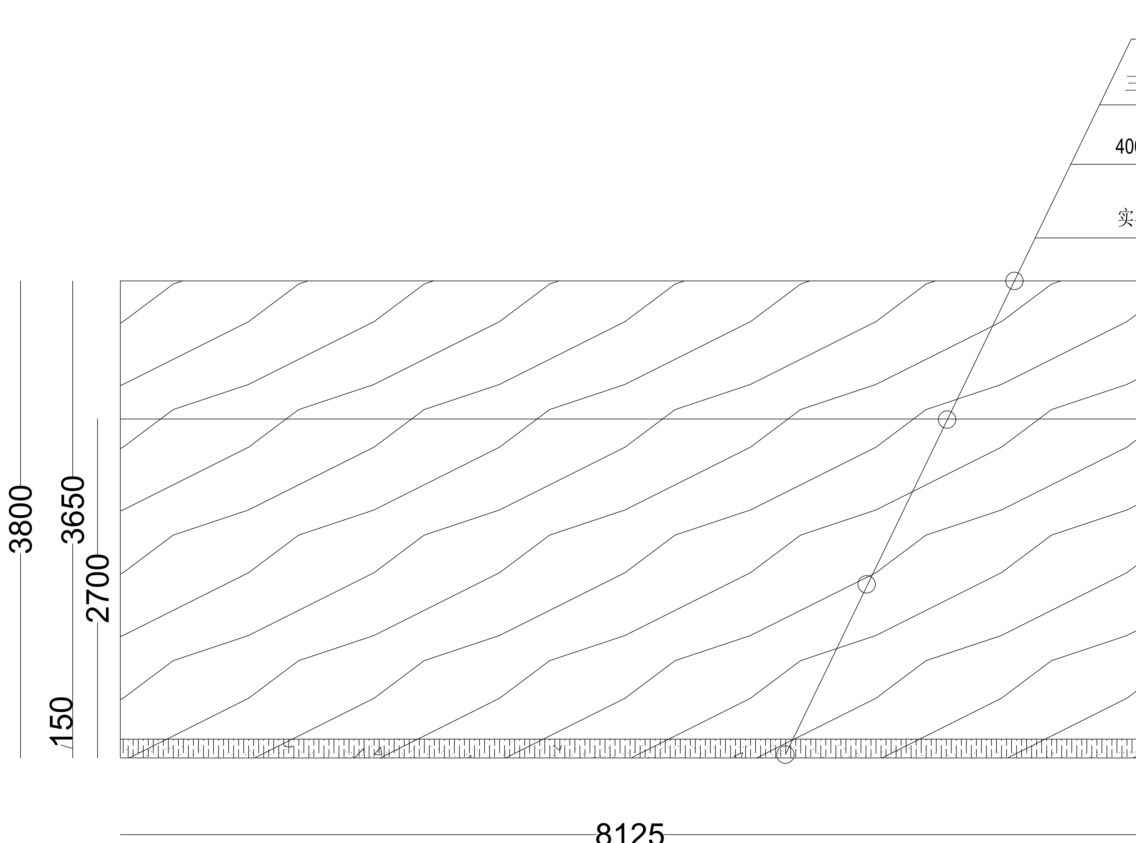
隔断断面图
